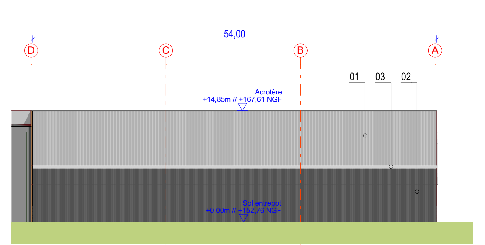
Plan de Façade Nord en file 11 - Entrepôt
